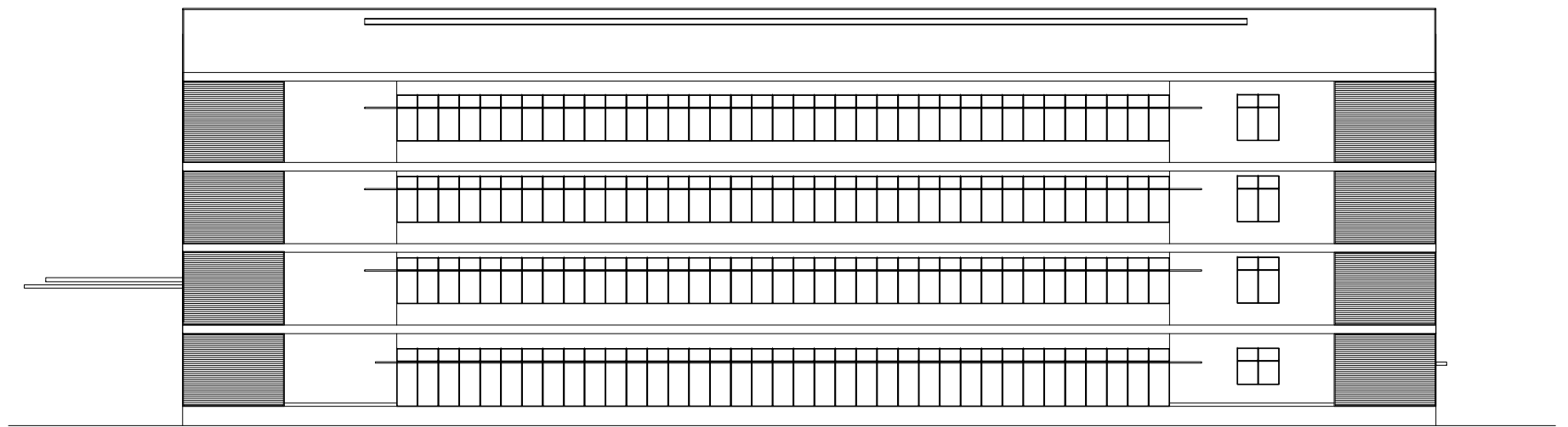
南立面図
