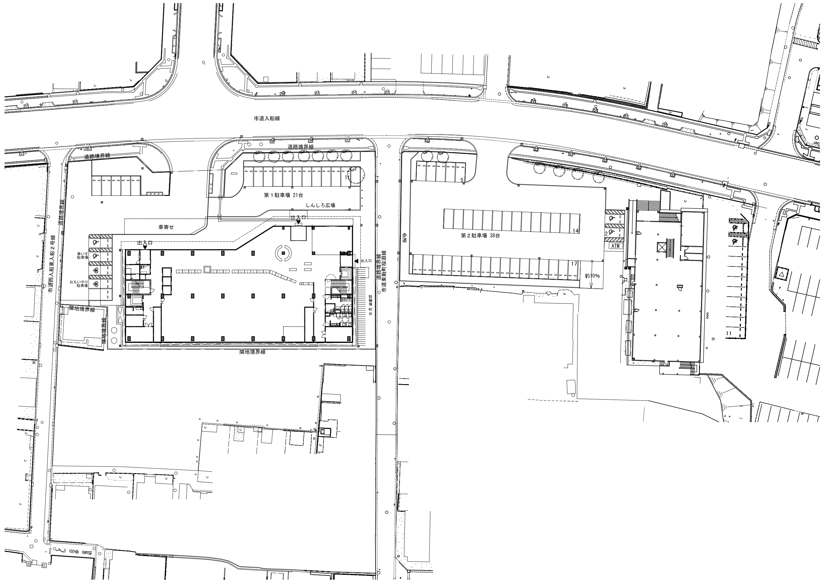
配置図兼外構計画図 1/600 (A3)
