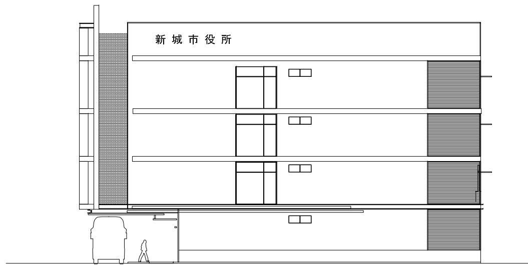
西立面図
