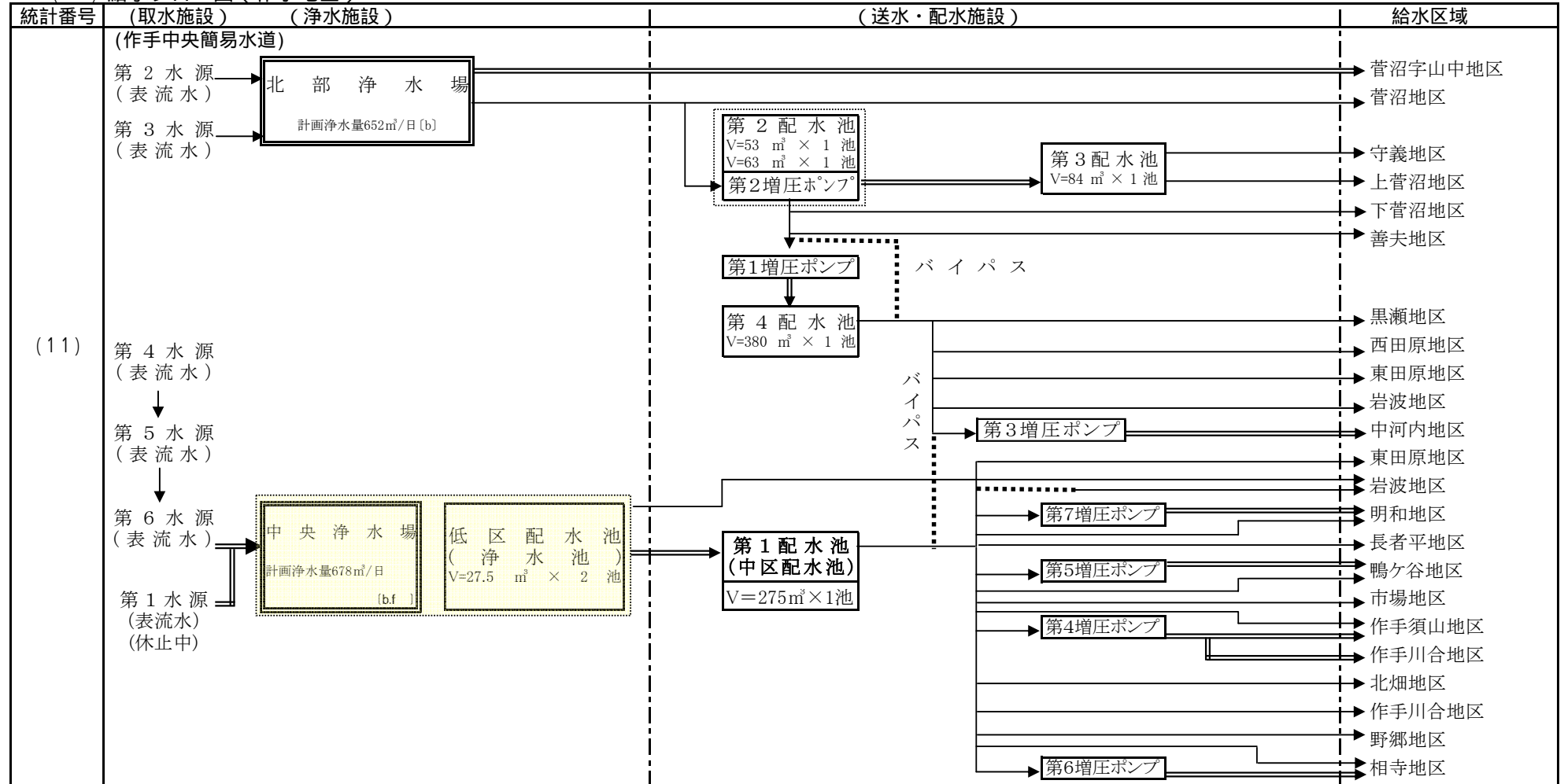
(14) 給水フロー図 (作手地区)
